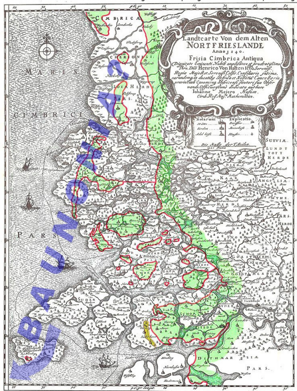
Nordfriesland um 1240 nach Johannes Mejer (1649) Küsten- und Inselkonturen von 2019 nach Angaben von Dipl. Ing. Hans-Peter Balfanz, Hamburg.
